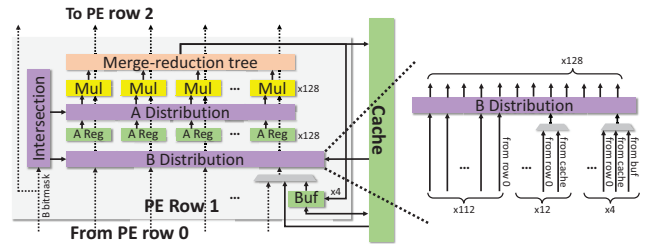
Fig. 6: PE row microarchitecture.
